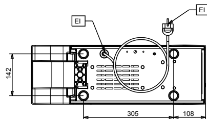
Boven aanzicht
